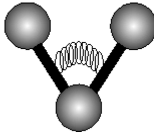
Ozonformel: O_3
